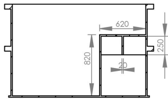
KESIT A-A
