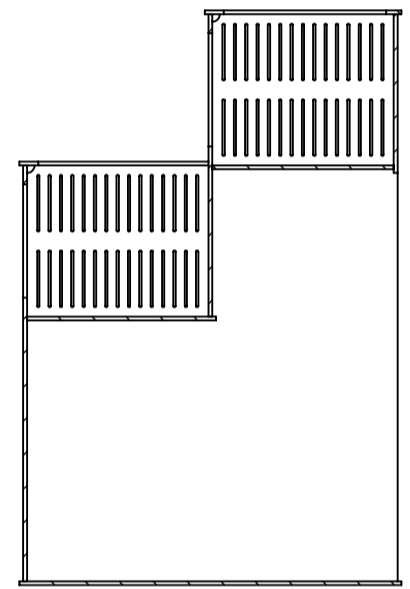
KESIT A-A
